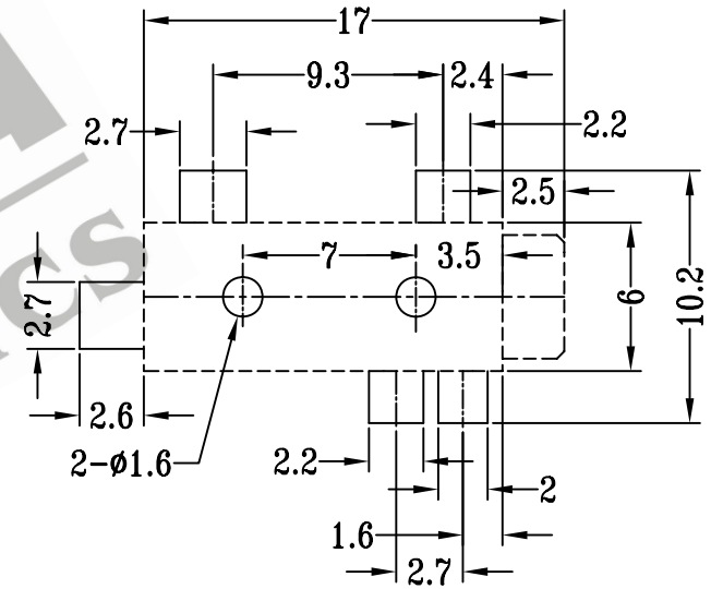
P.C.B LAYOUT
